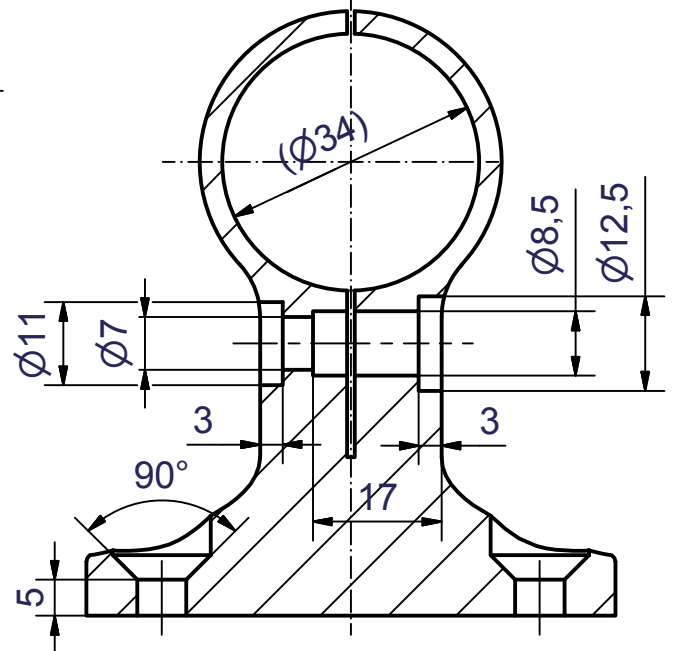
A-A (Darstellung ohne Schraube+Hülsenmutter)
